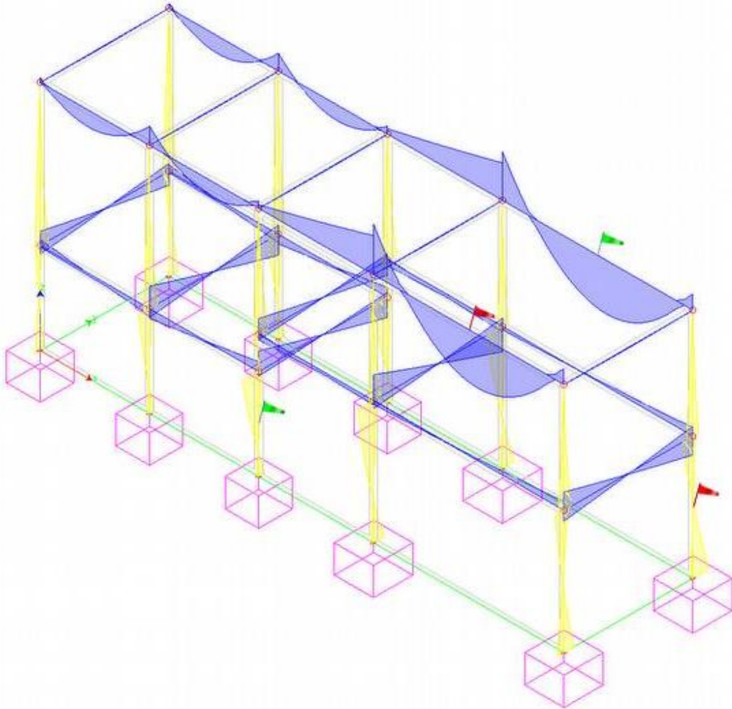
Figura 9: Involuppo dei momenti flettenti
