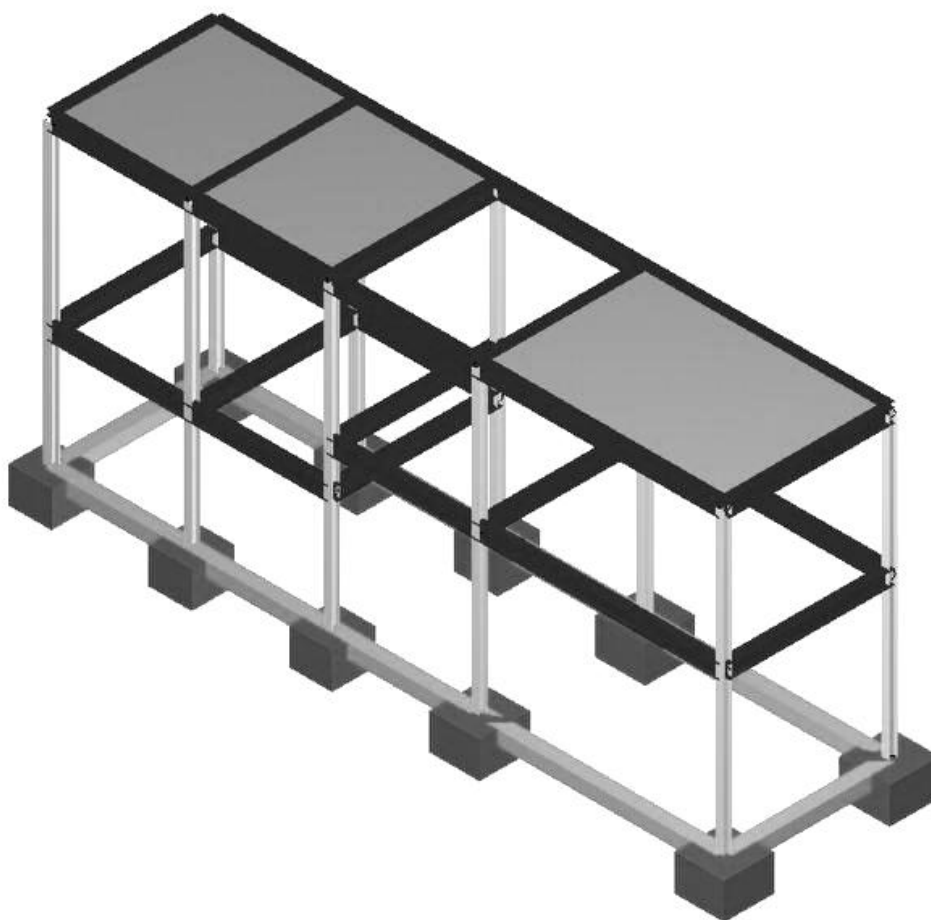
Figura 2 Modello tridimensionale della struttura del condensatore e della scala di accesso
