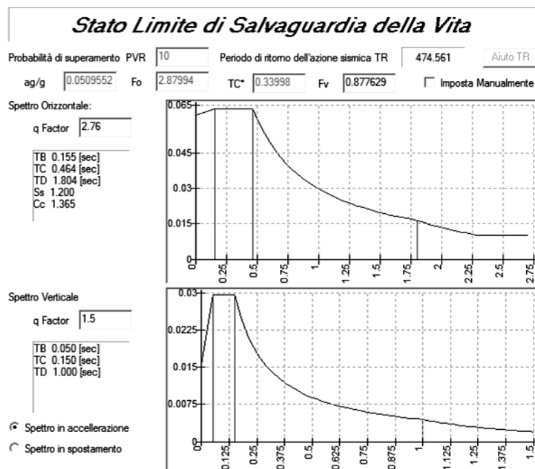
Figura 5: Spettri di calcolo agli SLV
