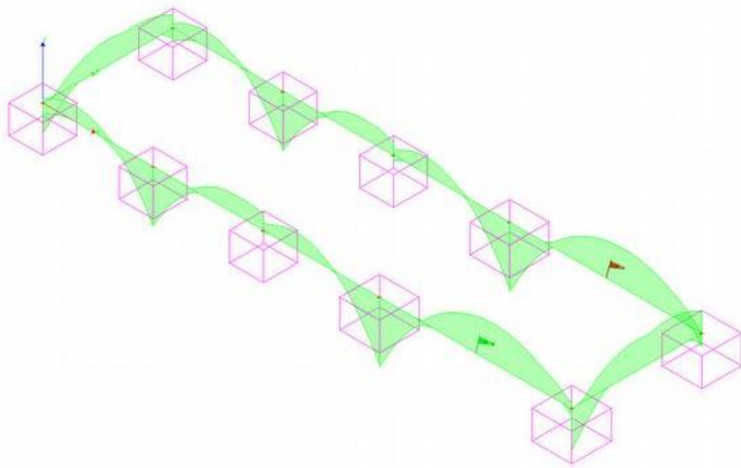
Figura 6: Involuppo delle pressioni sul terreno
