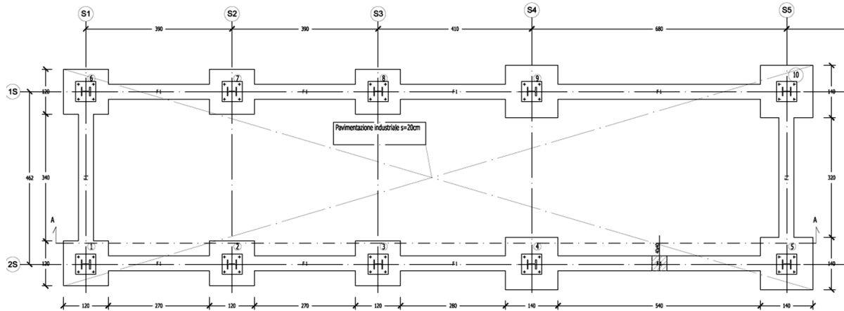
Figura 3 Pianta delle fondazioni del condensatore
