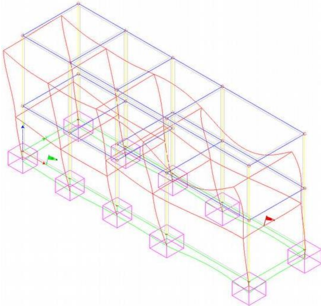
Figura 8: Spostamenti degli elementi per la combinazione SLU2
