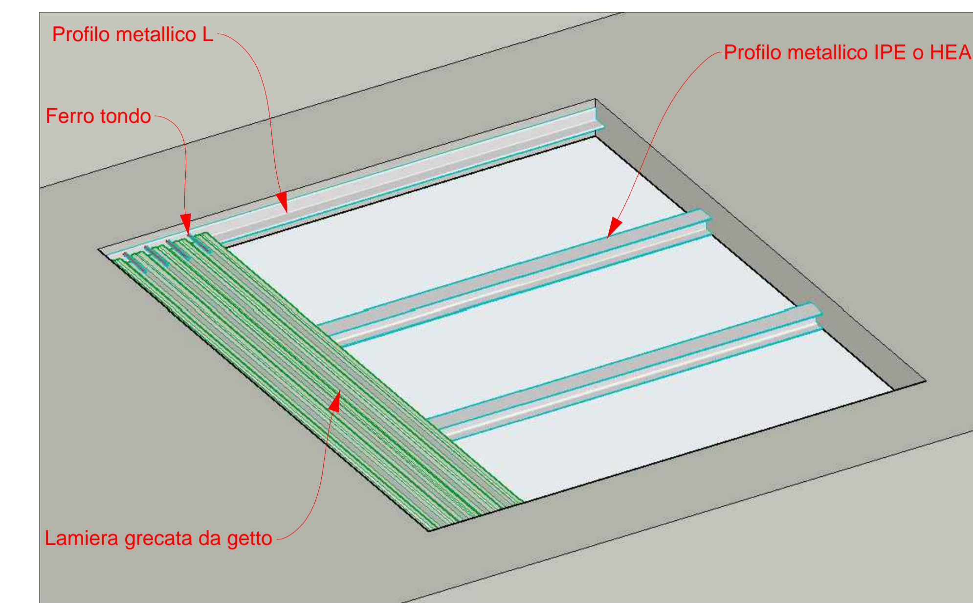
Particolare chiusura tramoggia
