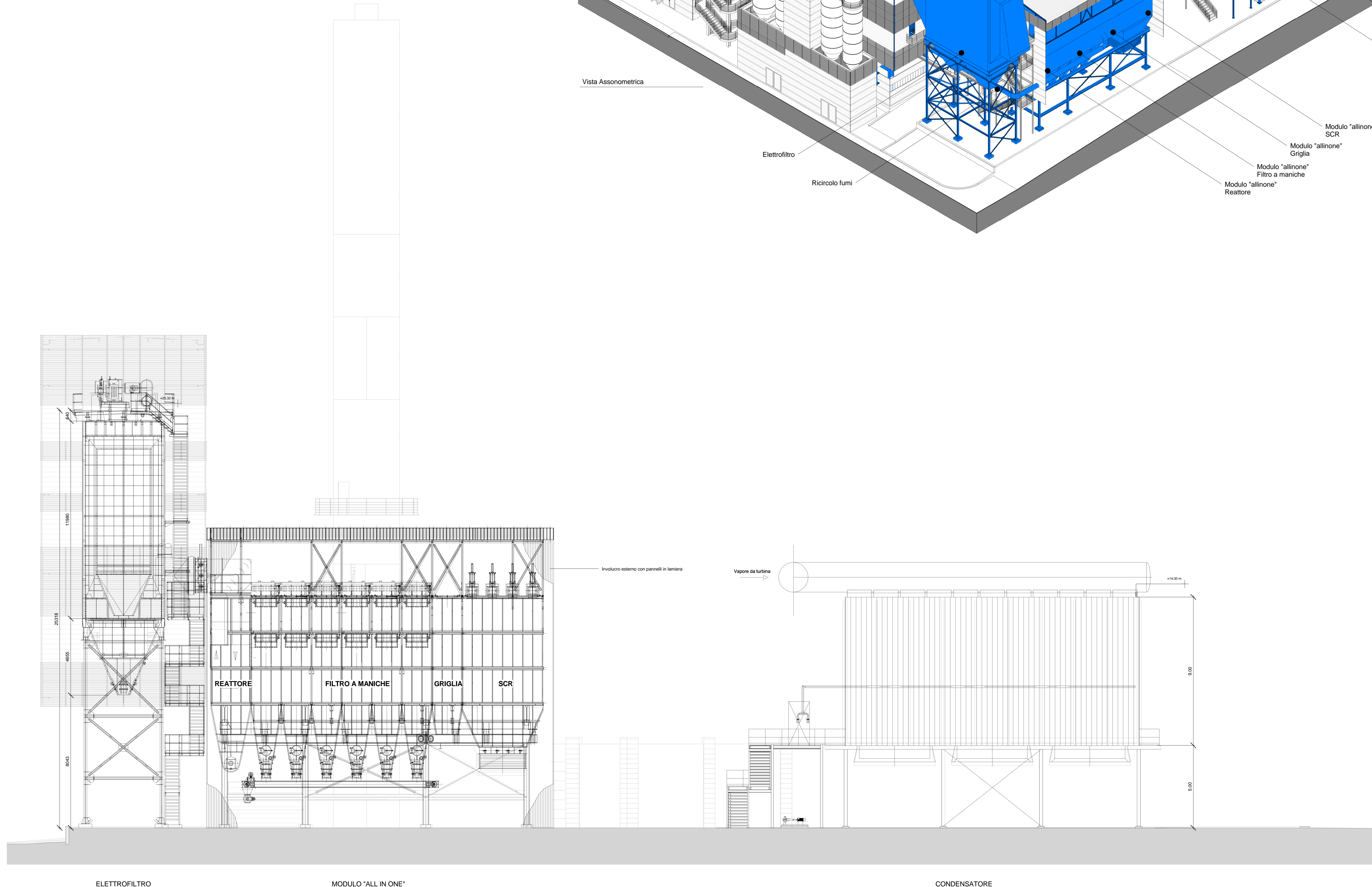
Sezione Longitudinale B-B
