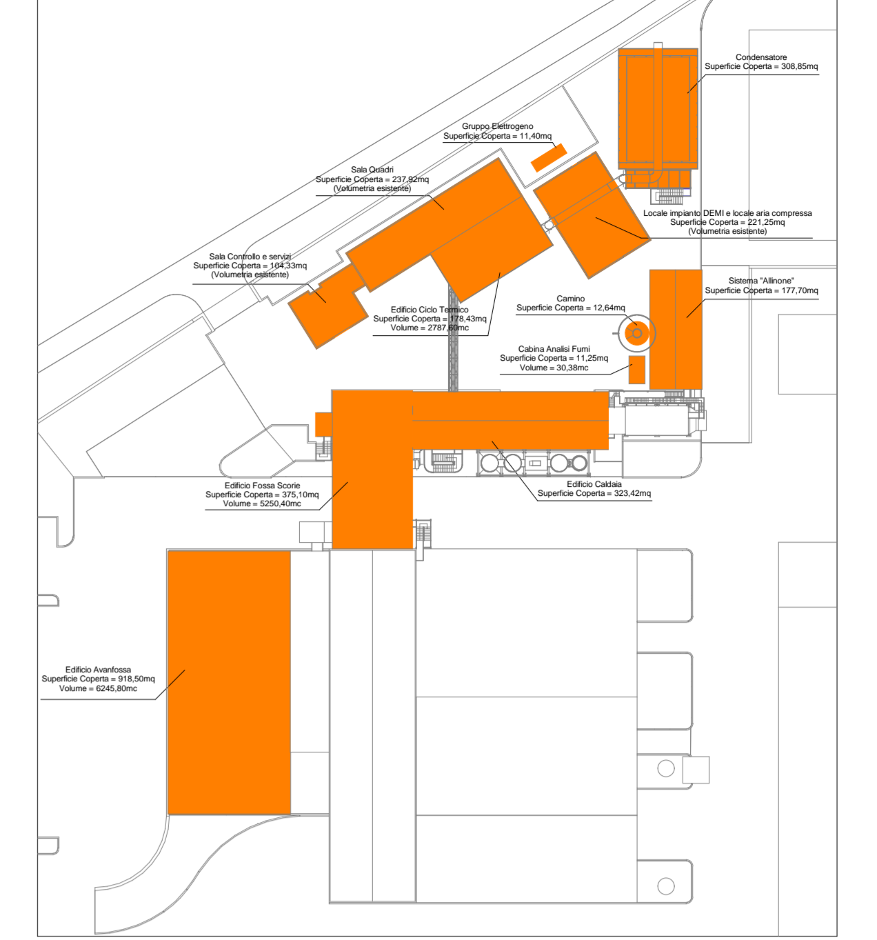
Calcolo delle superfici coperte e dei volumi di progetto
