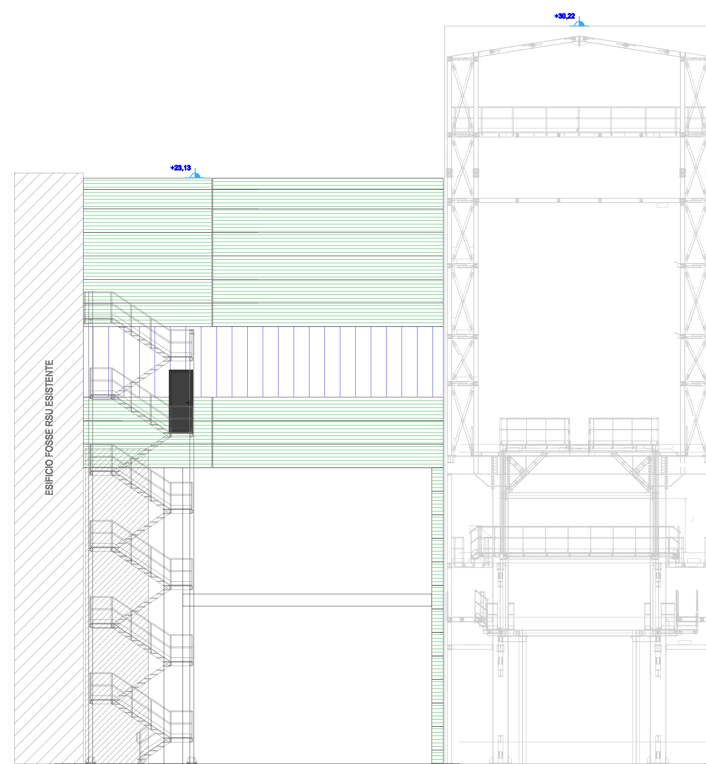
VISTA D – STATO DI FATTO
