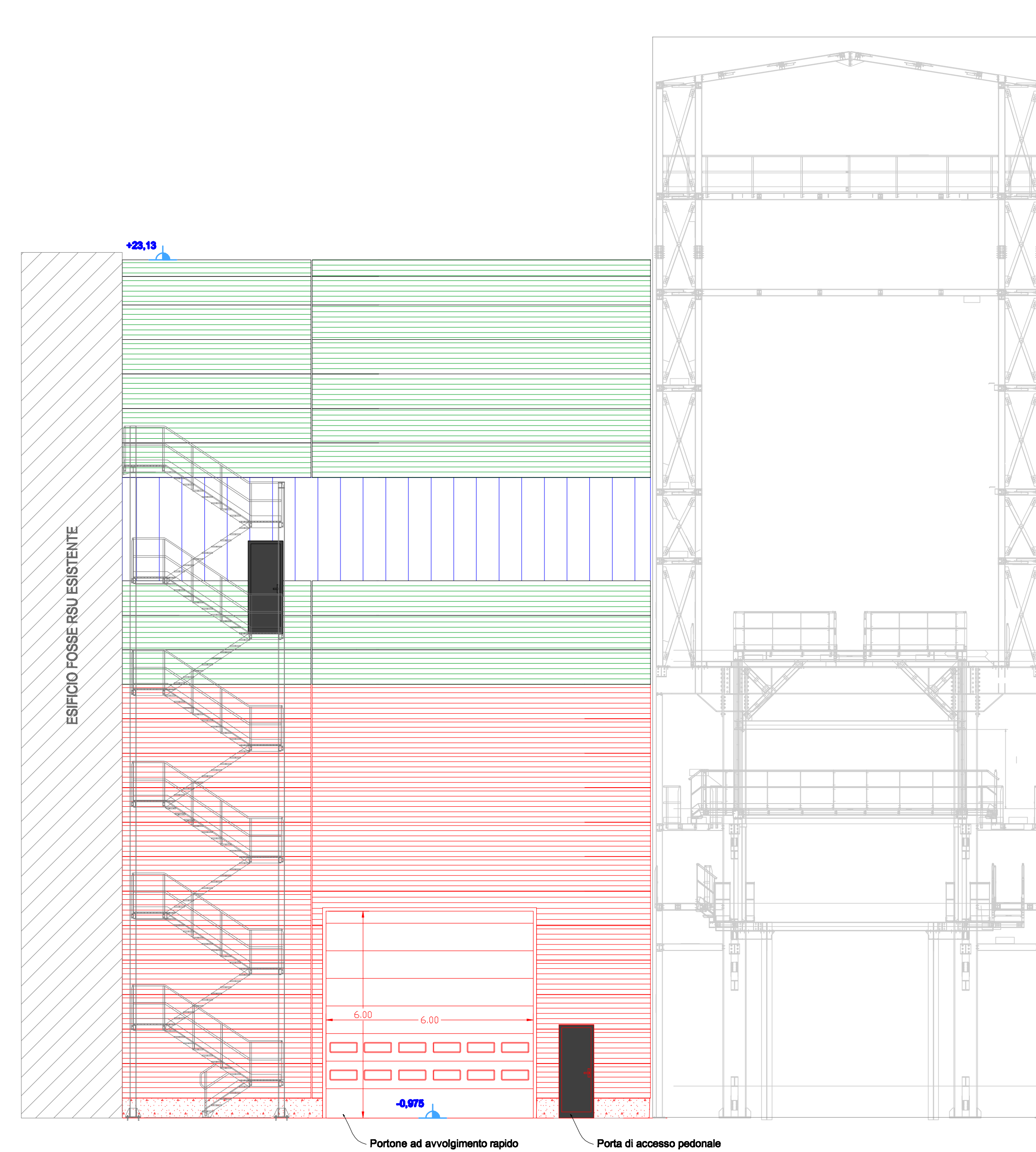
VISTA D – STATO VARIANTE
