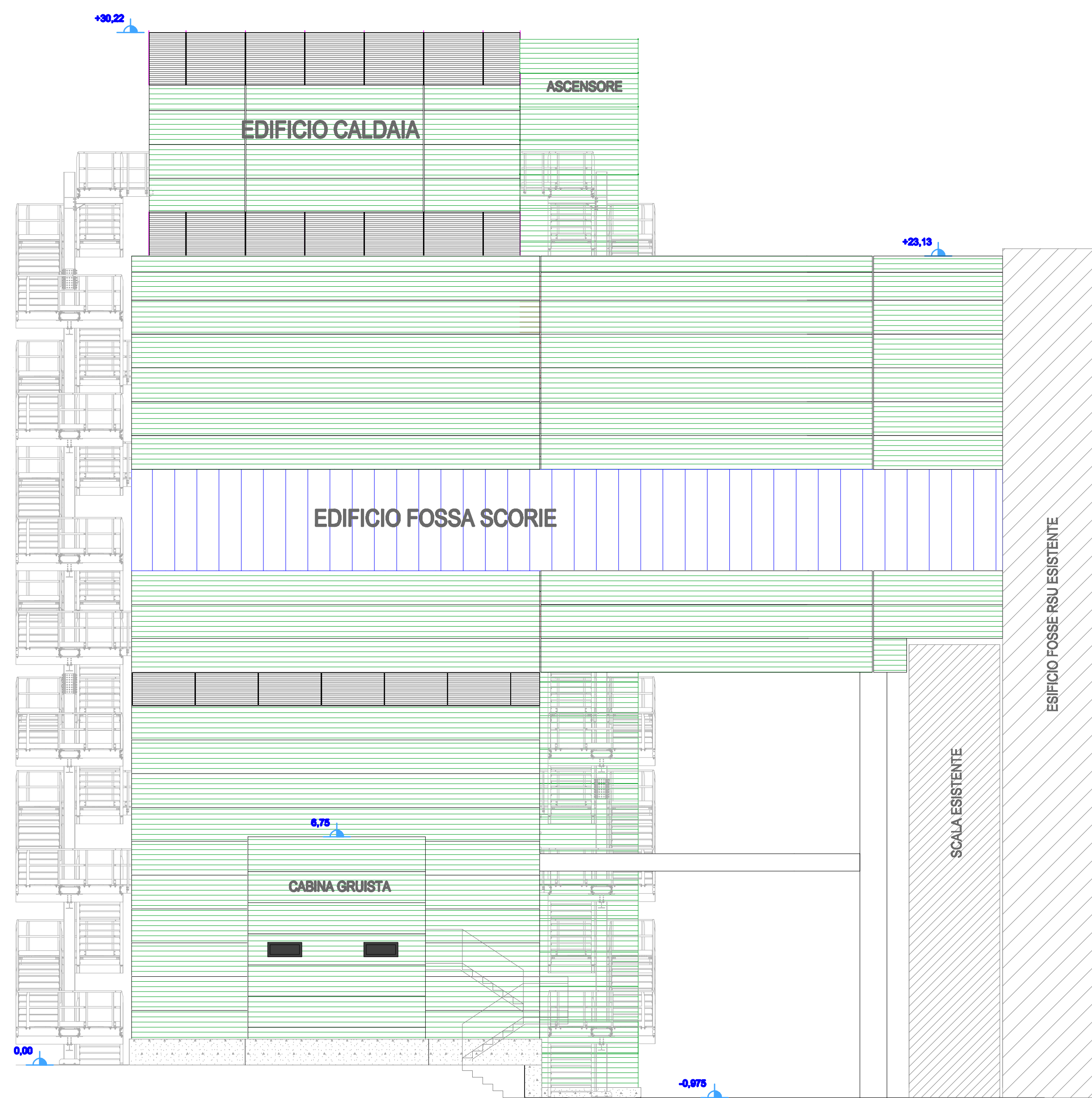
VISTA C – STATO DI FATTO
