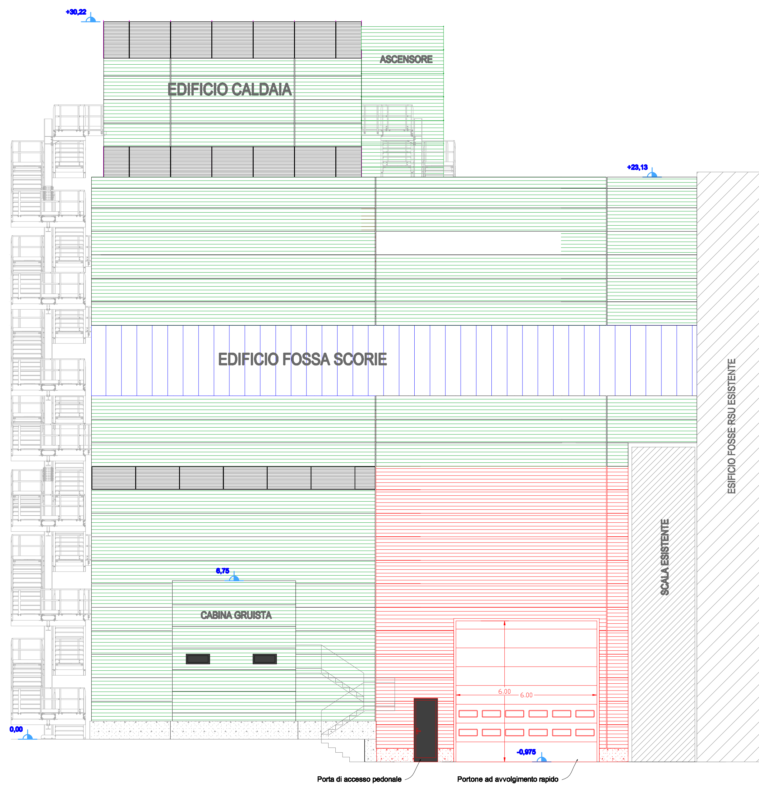
VISTA C – STATO VARIANTE
