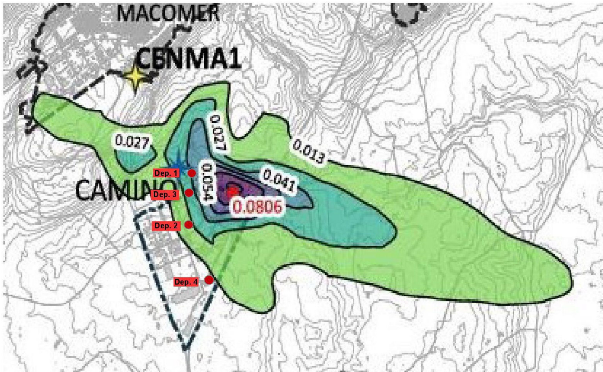
Schema punti di posizionamento dei deposimetri in relazione allo schema di diffusione degli inquinanti in atmosfera
